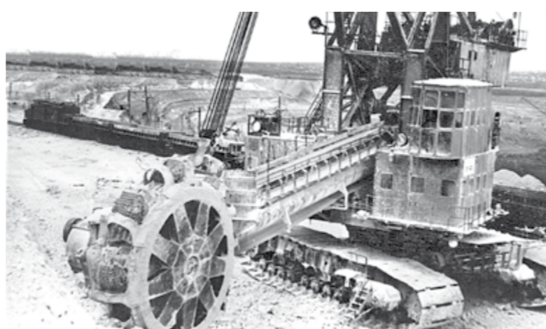
1970 год. Губкинский район. На Лебединском руднике роторный экскаватор ведёт вскрышные работы с одновременной погрузкой породы в думпкары
