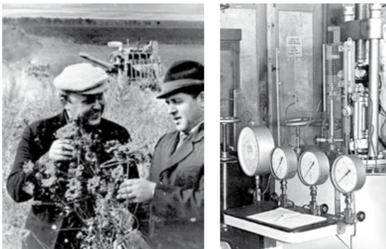
1973 год. Прибор стабилометр СВД-4 разработан Белгородским институтом ВИОГЕМ для определения деформационных, прочностных и фильтрационных свойств горных пород
